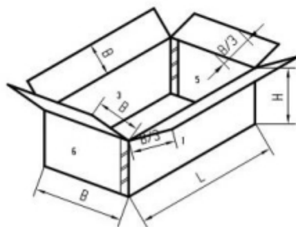
法兰球铁球阀包装箱 Q41F-16QA-X01
